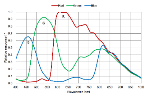
MV-CS032-10GC 量子效率
