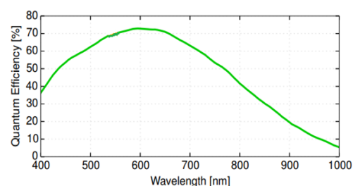
MV-CS032-10GM 量子效率
