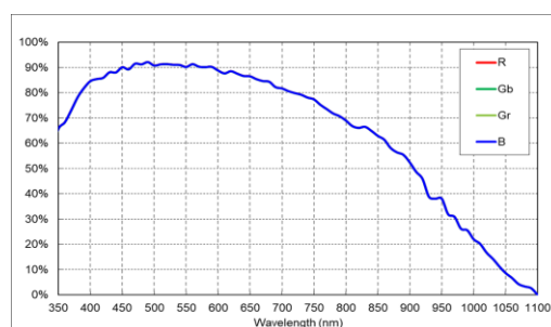
MV-CS020-60GM V5 量子效率
