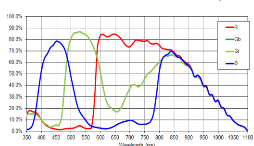
MV-CS020-60GC V5 量子效率
