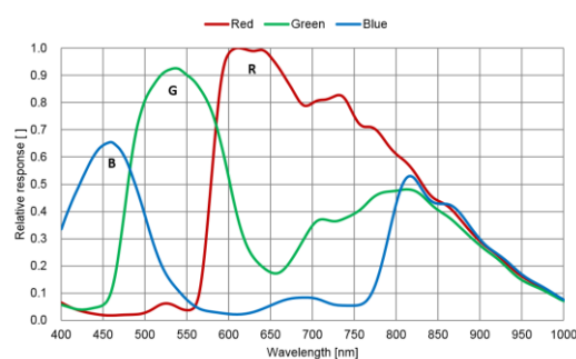
MV-CS050-10GC V5 量子效率
