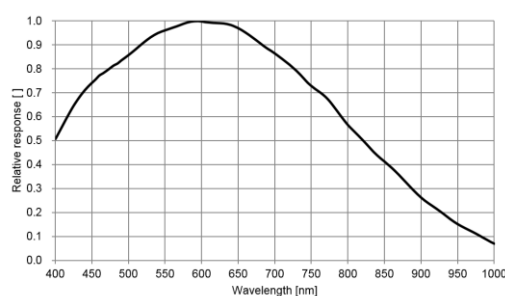
MV-CS050-10GM V5 量子效率
