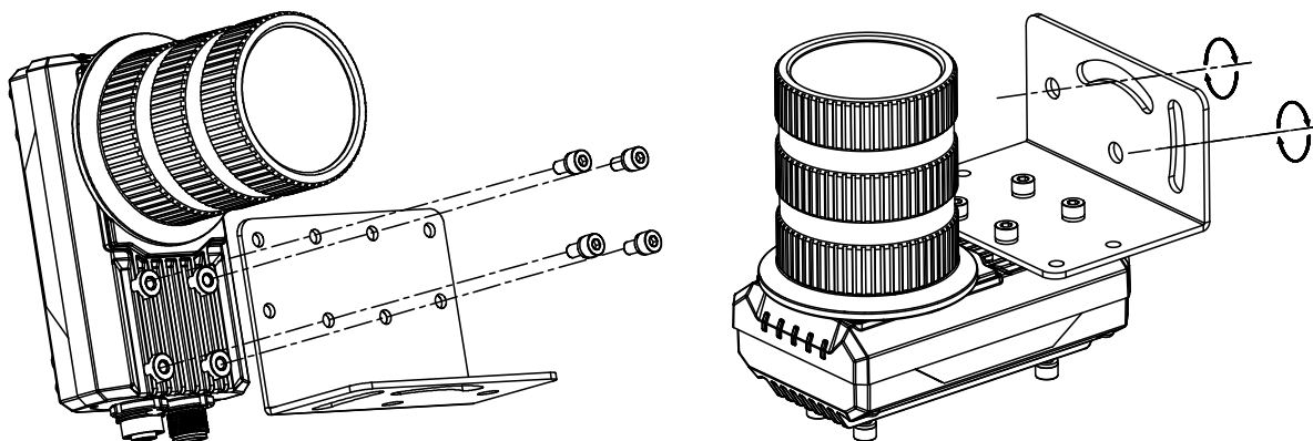
图3-2 正面安装
